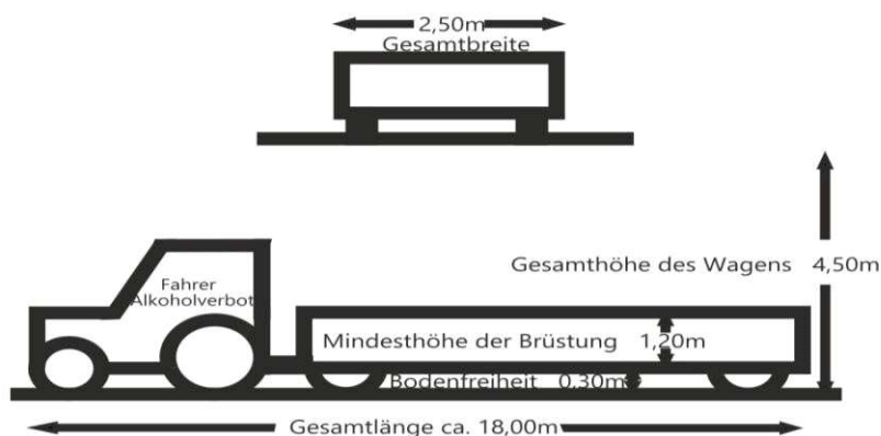
Abmessungen der Wagen, für die Wagenbauer
